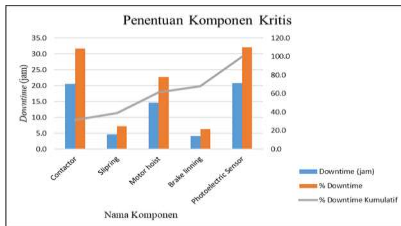
Gambar 3. Diagram Pareto Penentuan Komponen Kritis
